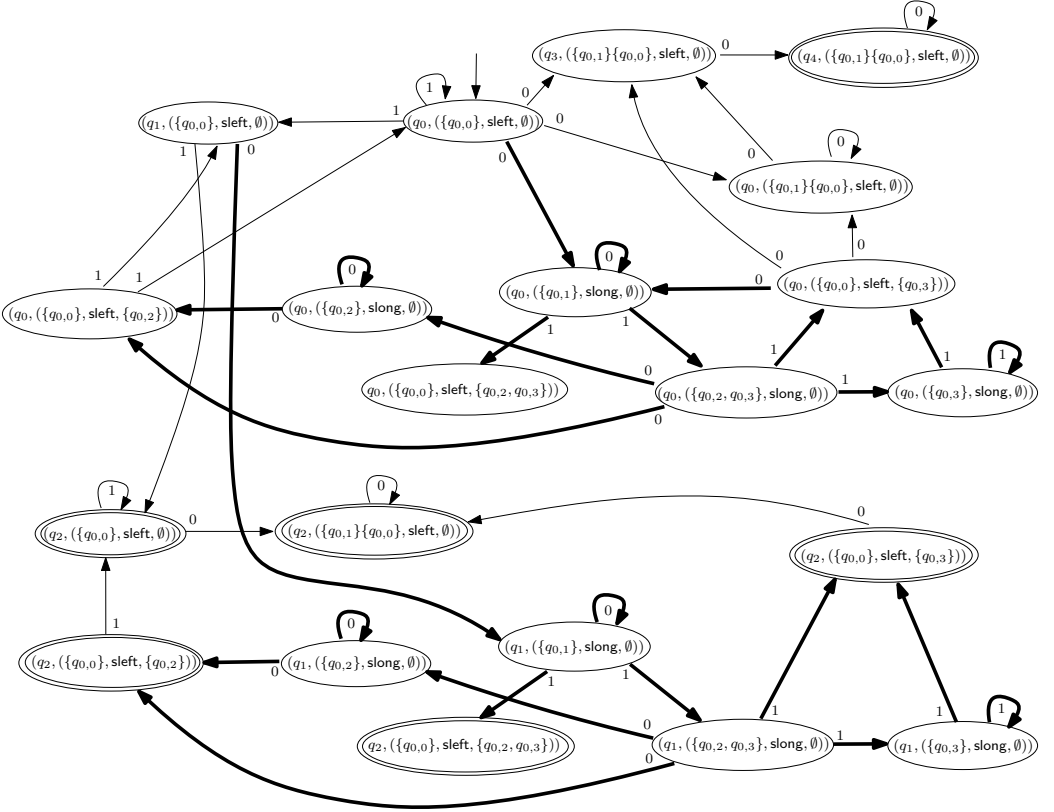
Fig. 9. The NFA \mathcal{B}_{\mathcal{A}_1, e_0, T_z}
